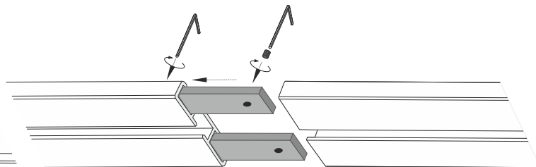
Łączenie profili pojedynczych
