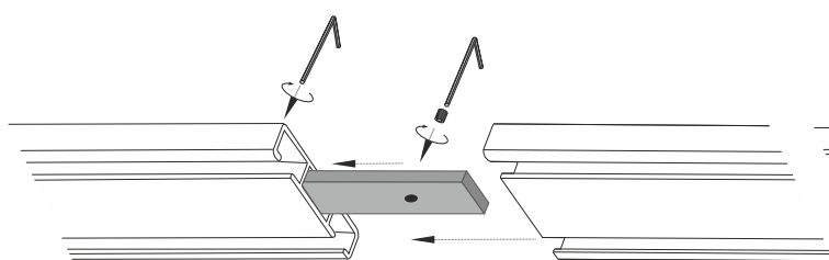
Łączenie profili podwójnych
